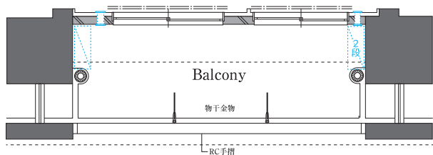
2~4階手摺形状
